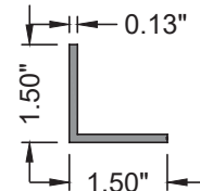
ALU-A-019 ANGLE ALUM. 6063-T6
