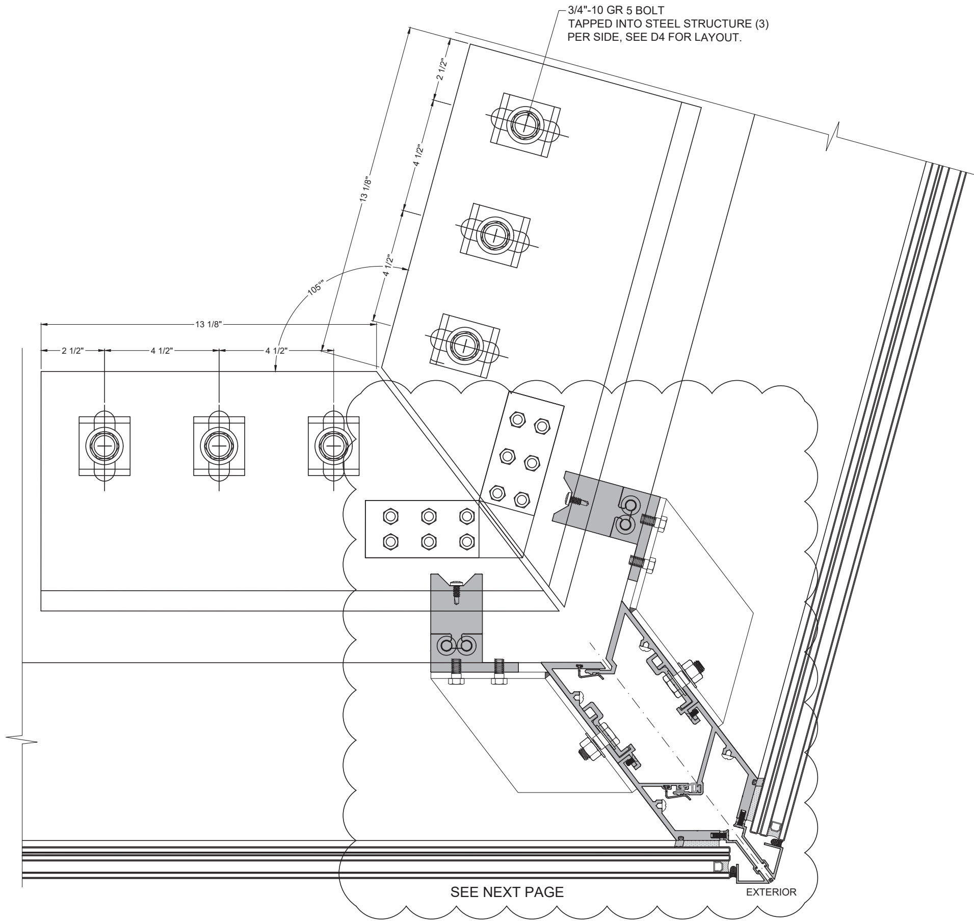
1 DETAIL D13 105° CORNER
