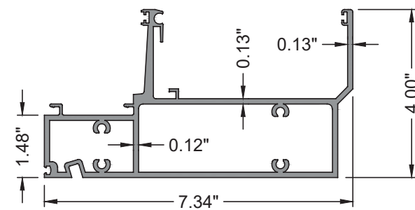
E37 GW-7000-154 HORIZONTAL ALUM. 6063-T6
