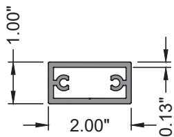
E39 103-047 JAMB SPACER ALUM. 6063-T6
