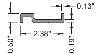
E33 GW-7000-143 SPLICE ALUM. 6061-T6
